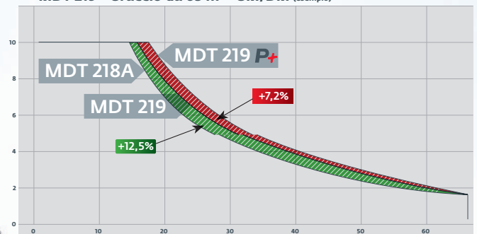
MDT 219 – braccio da 65 m – SM/DM (esempio)
