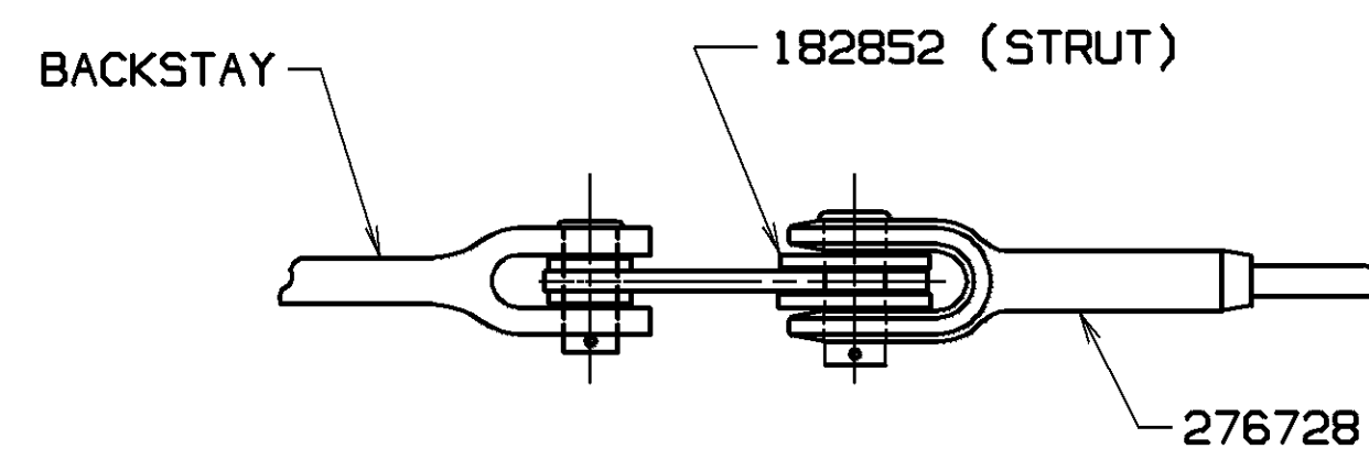
VIEW A-A
