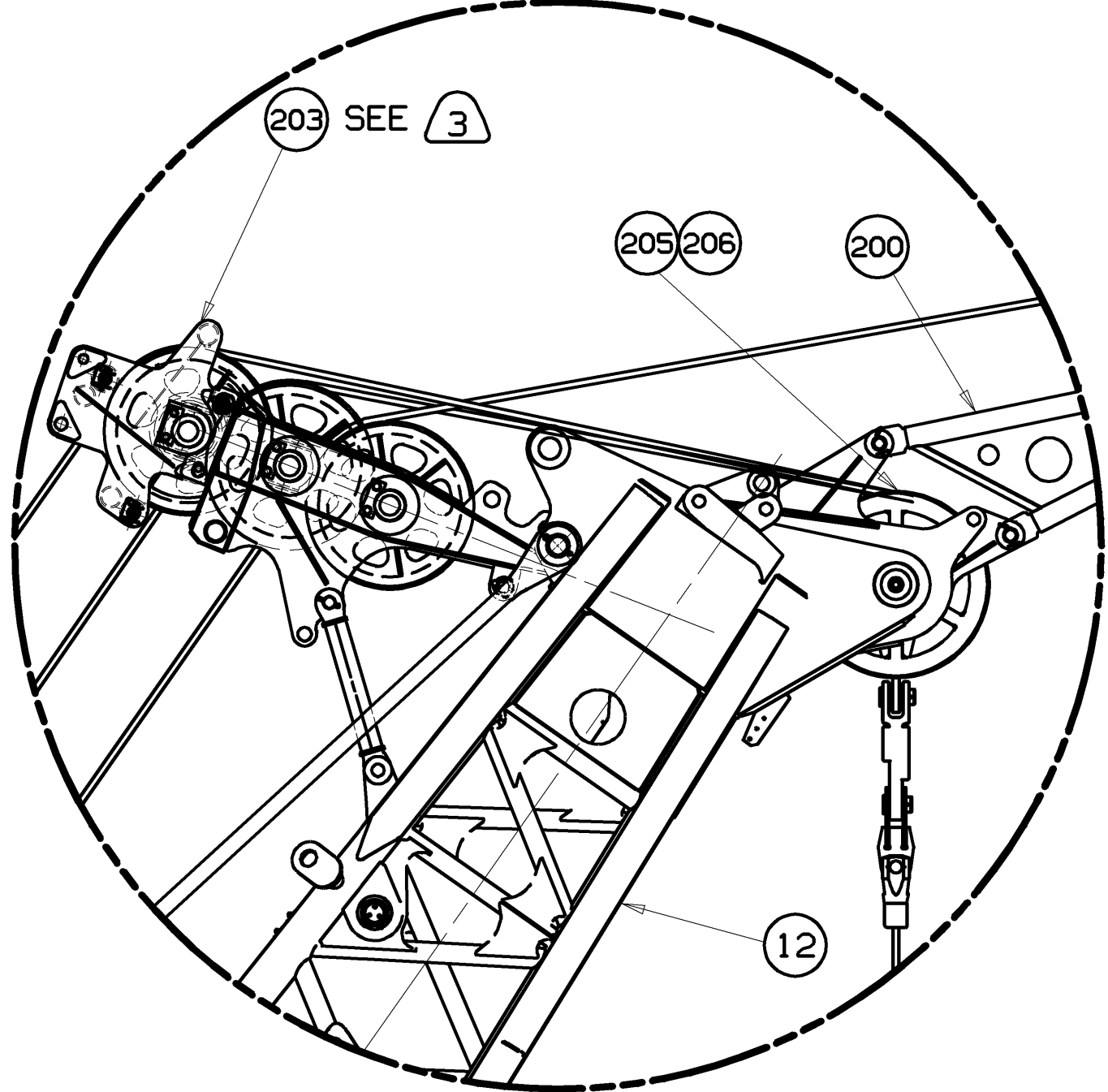
DETAIL "A" SCALE: 0.04
