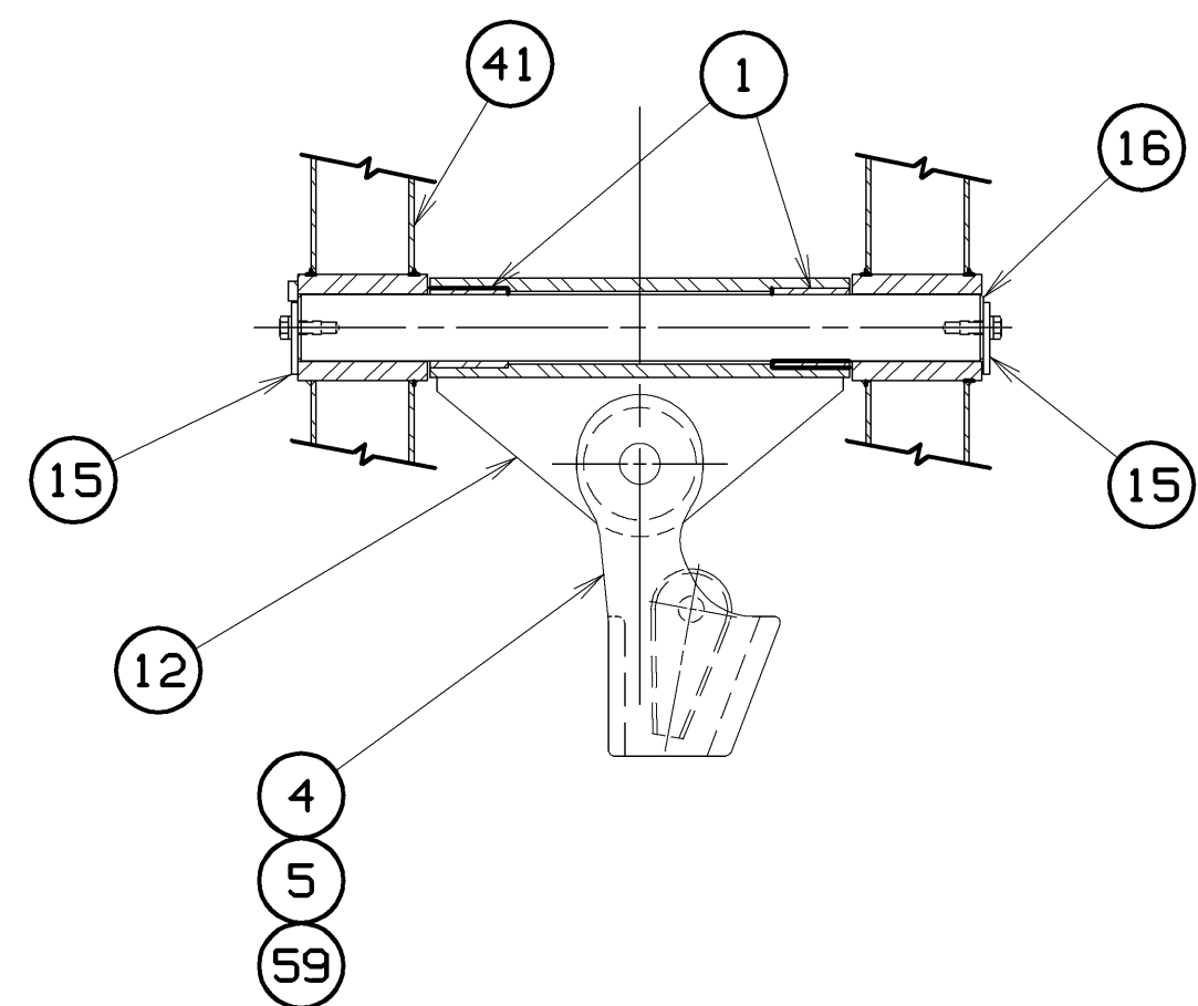
SECTION "F" - "F" SCALE: 1.50=1FT.
