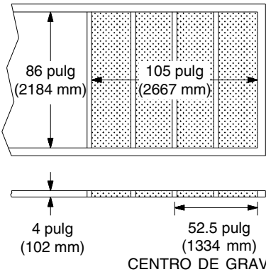
CONTRAPESO DE PLATAFORMA PARA 3000 lb (1360 kg)
