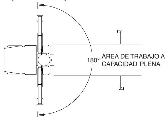
DIAGRAMA DE ÁREA DE TRABAJO
