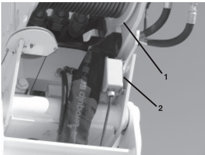
Ubicación de caja de empalmes de ángulo mínimo
