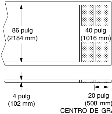
CONTRAPESO DE PLATAFORMA PARA 1150 lb (520 kg)
