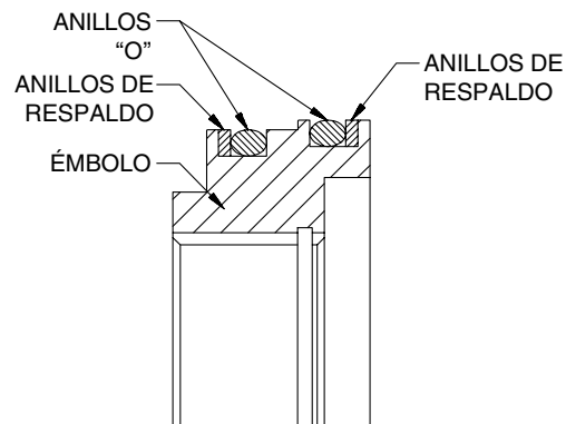
INSTALACIÓN DE ANILLOS "O"
