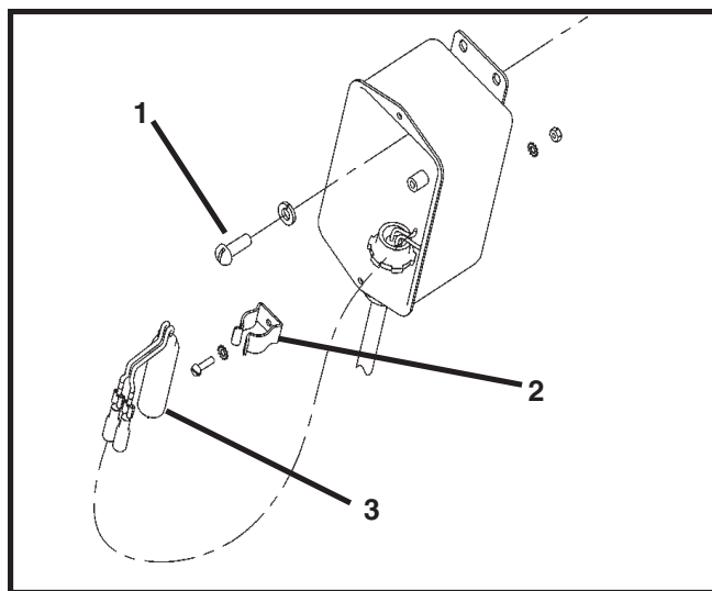
Ajuste de interruptor de ángulo mínimo
