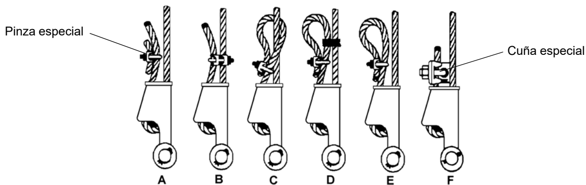
Receptáculo de cuña
