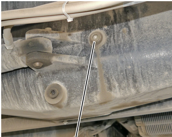
Tapón de llenado/revisión de la caja del eje trasero
