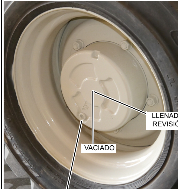
Tapón de llenado/revisión del cubo de la rueda
