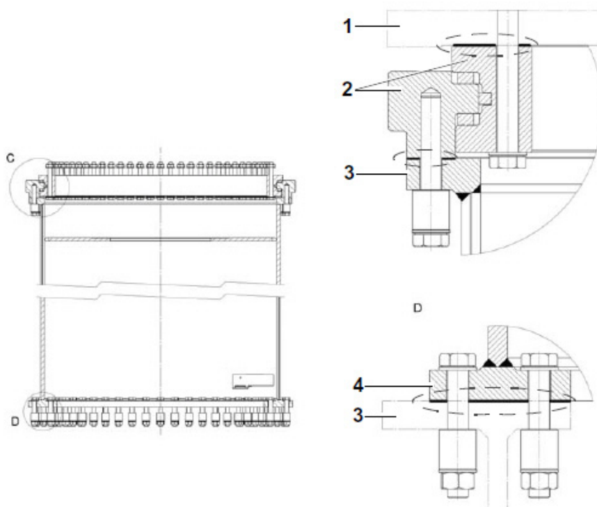
Conexión de brida con Loctite
