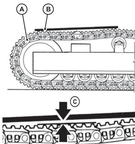
Fig. 25 Determinación de la tensión de cadena
