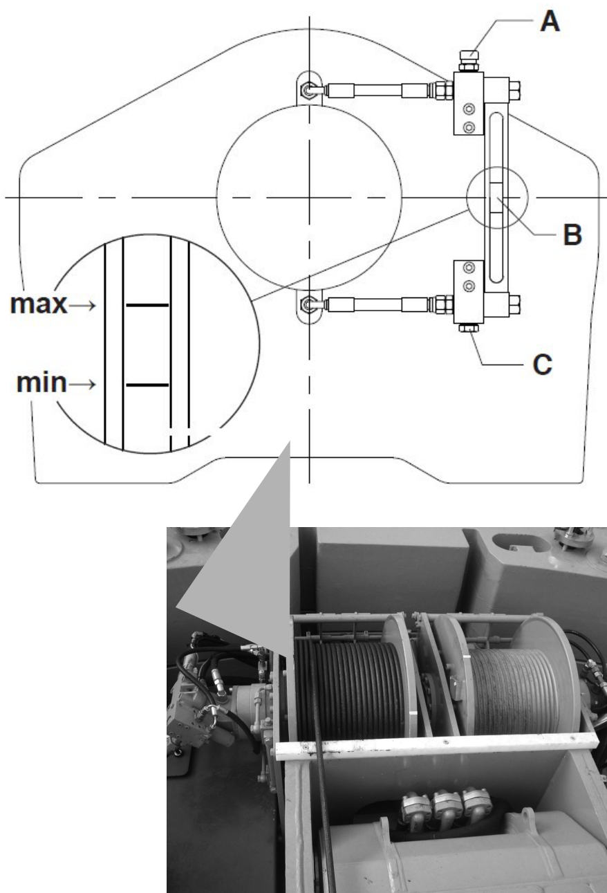
Fig. 23 Malacate
