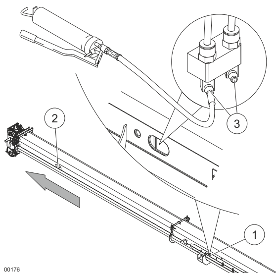
Fig. 37 Lubricación de la pluma telescópica
