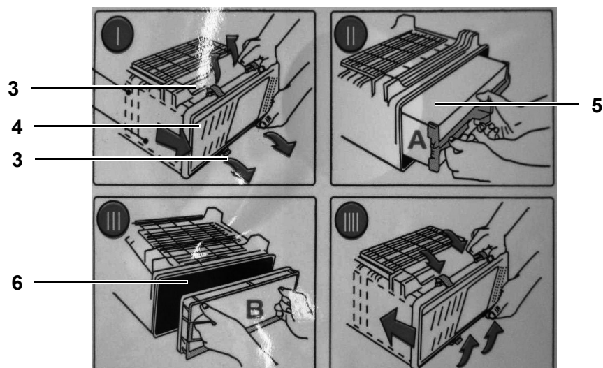
Fig. 10 Sustitución del filtro de aire
