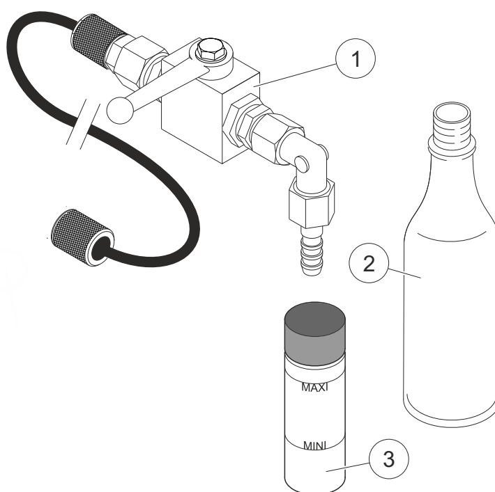
Fig. 3 Materiales para muestreo del aceite hidráulico
