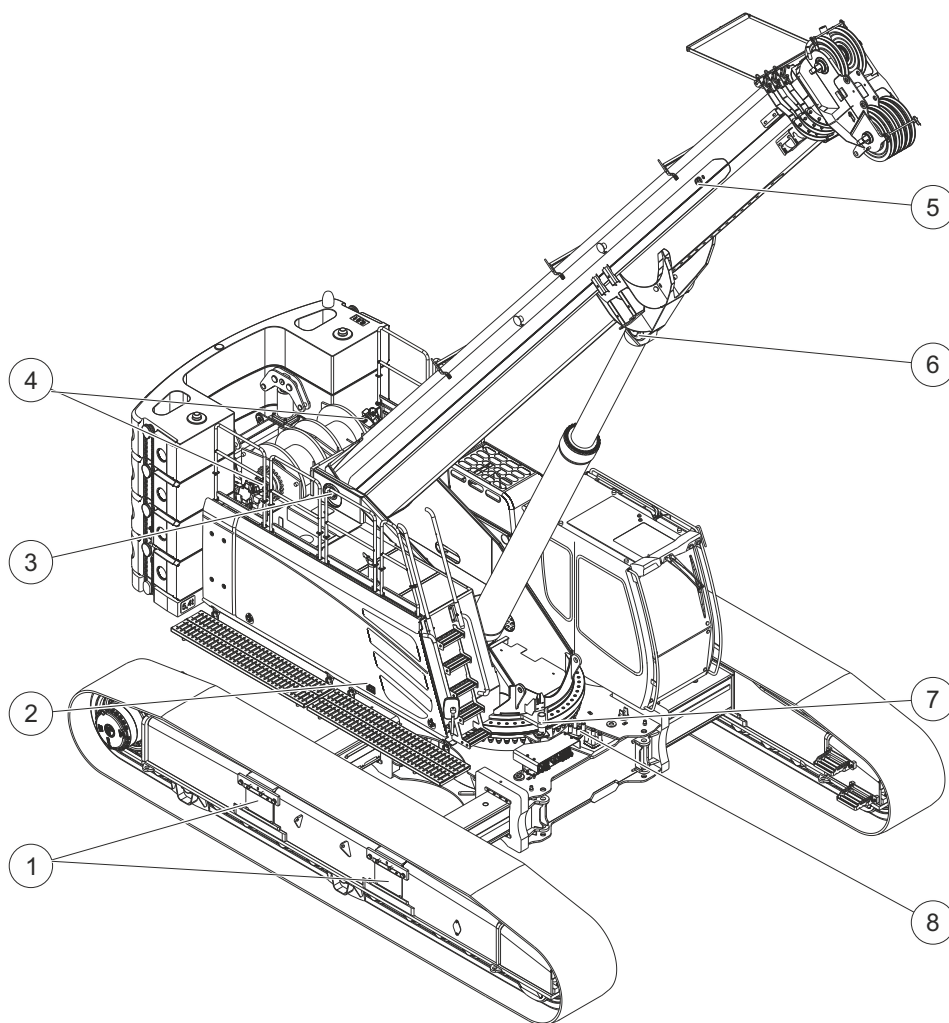
Fig. 6 Puntos de lubricación de la máquina
