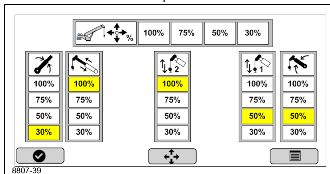
Salida N.º 3 de palanca de control
