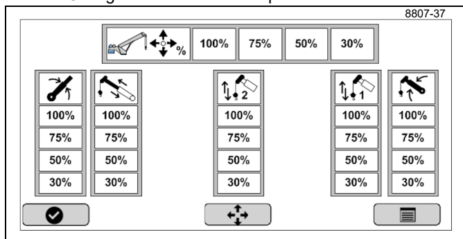
Configuración de salida de palanca de control
