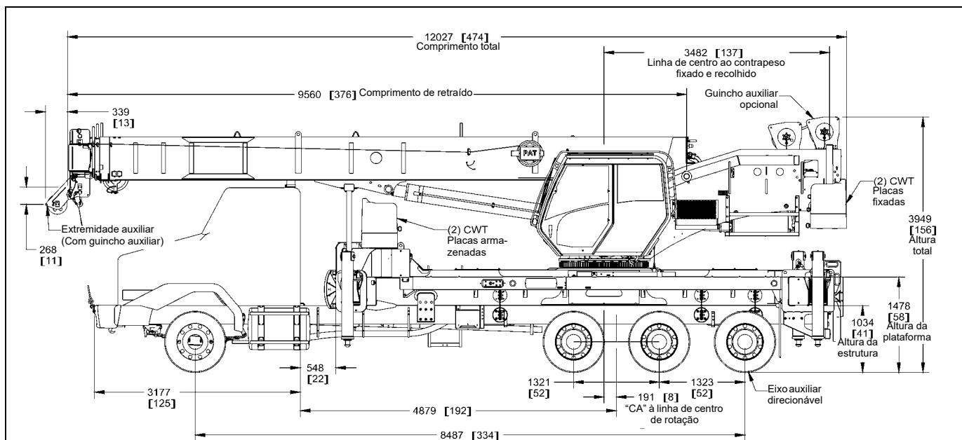
Desenho de layout mínimo do caminhão NBT55102
