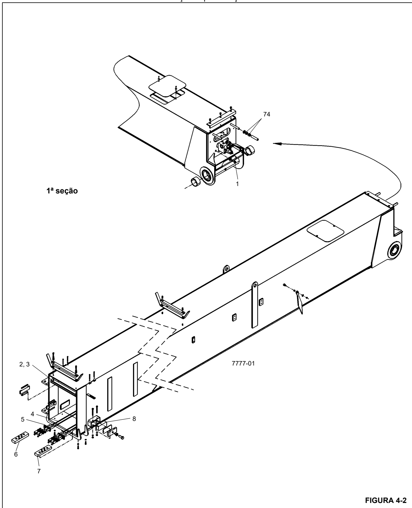
Lança de quatro seções
