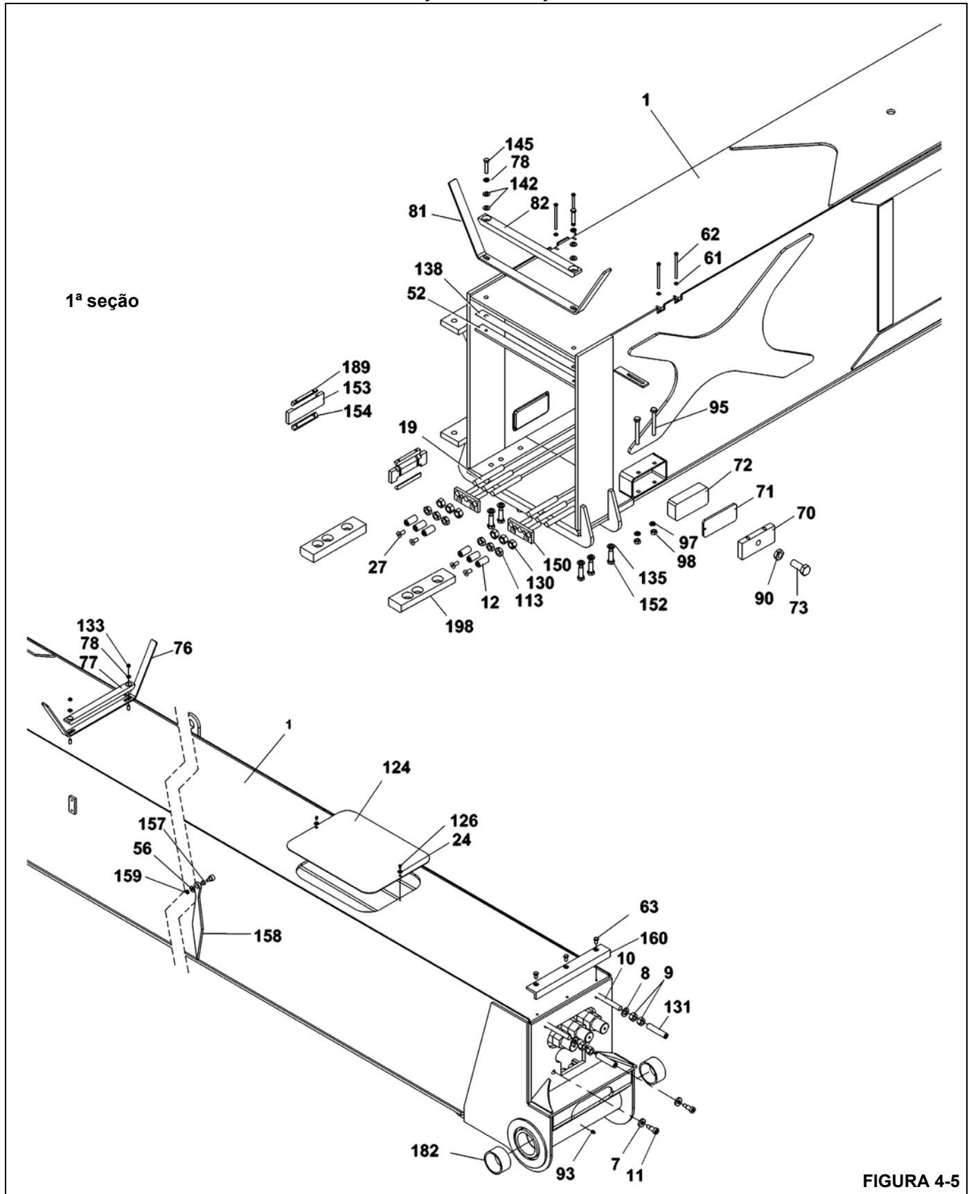
Lança de cinco seções
