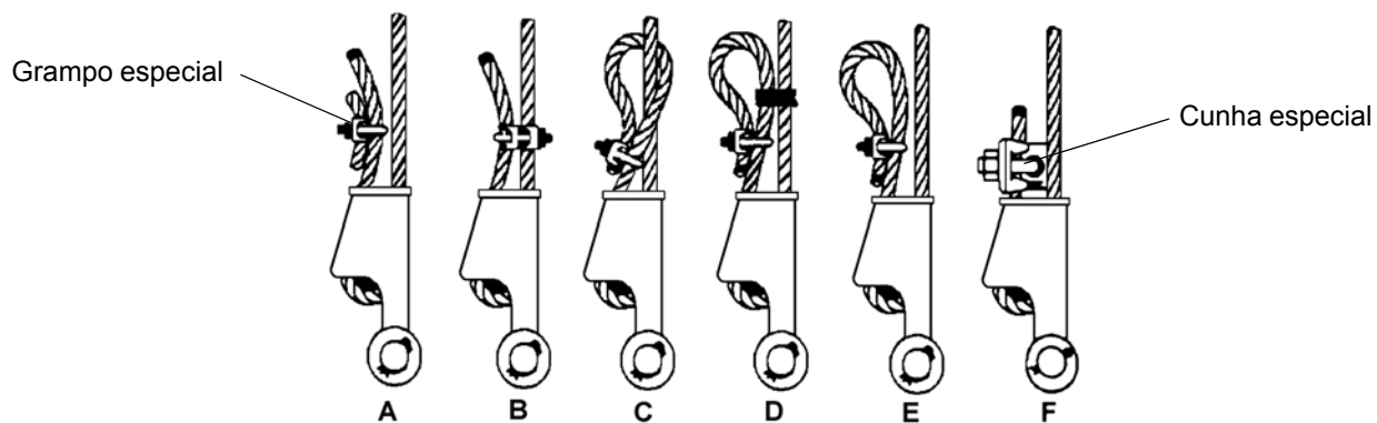
Terminal com cunha
