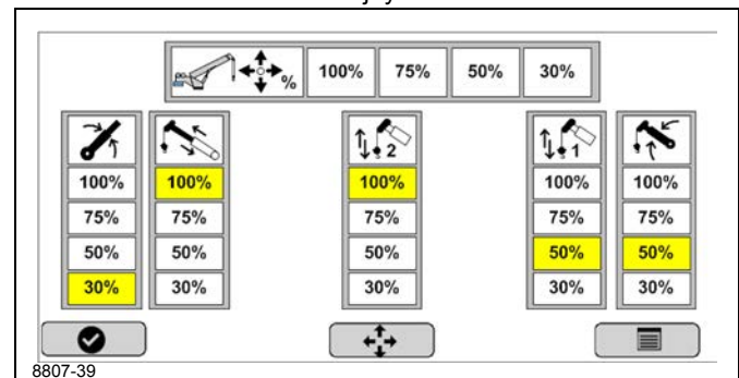
Saída do joystick nº 3
