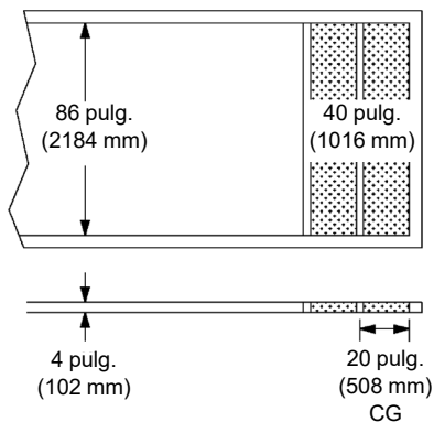
CONTRAPESO EN PLATAFORMA PARA 1150 LB (520 KG)
