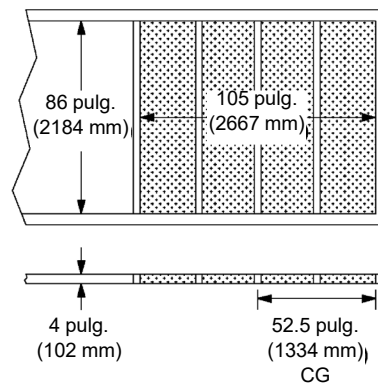
CONTRAPESO EN PLATAFORMA PARA 3000 LB (1360 KG)
