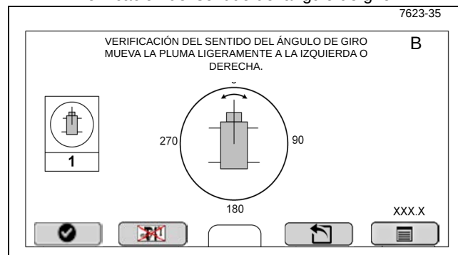
Verificación del sentido del ángulo de giro
