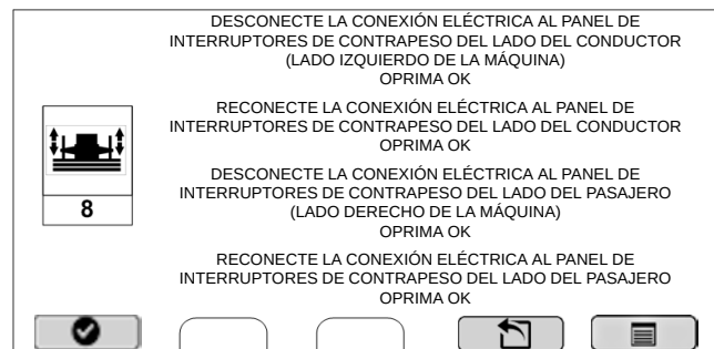
Calibración de tablero de interruptores de contrapeso
