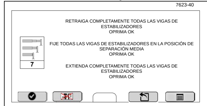
Calibración del sensor de longitud de estabilizador
