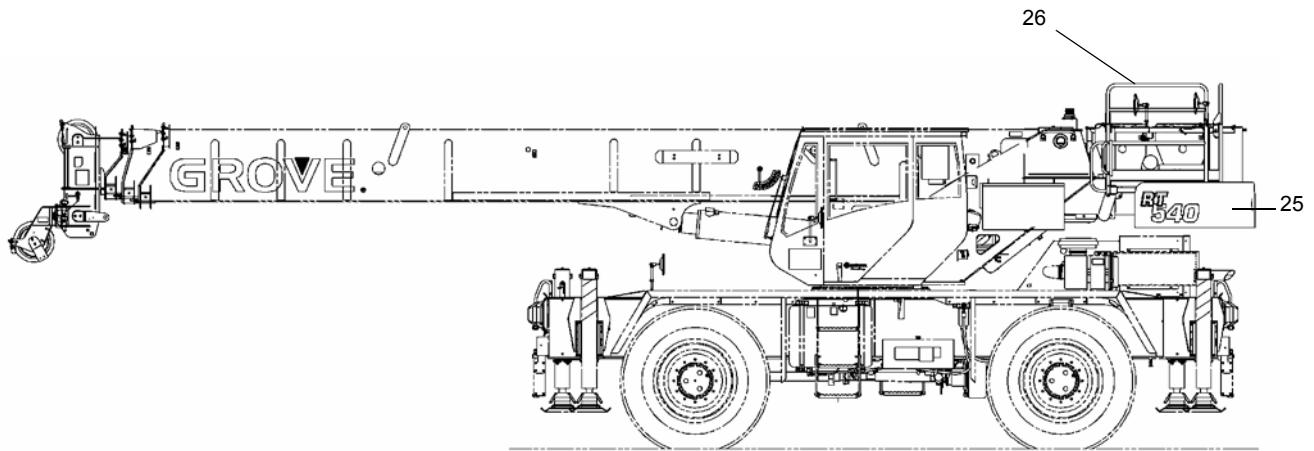
Vista lateral esquerda - Unidades de contrapeso fundido
