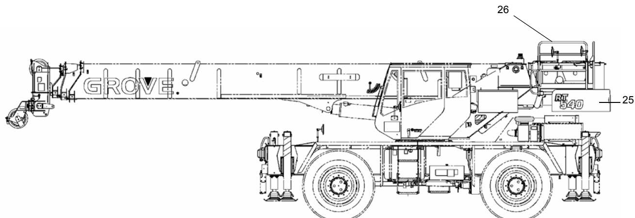
Vista izquierda - Máquinas con contrapeso fundido
