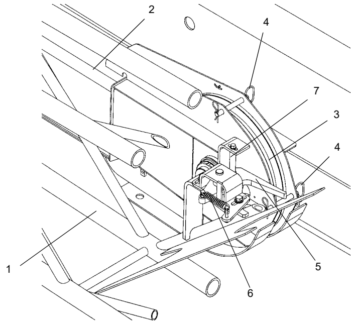
DETALLE E
