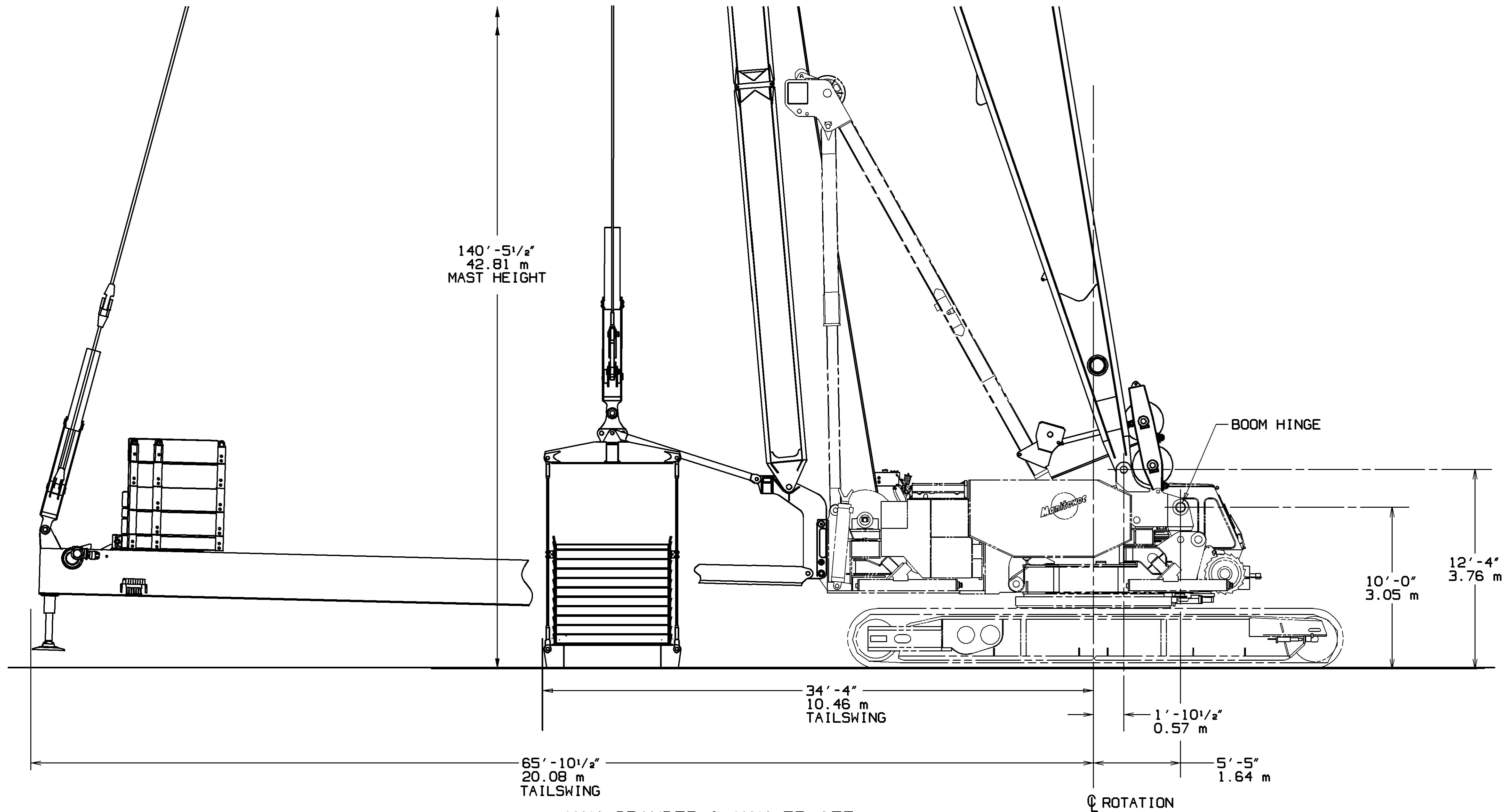
MAX-SPANDER & MAX-ER 175
